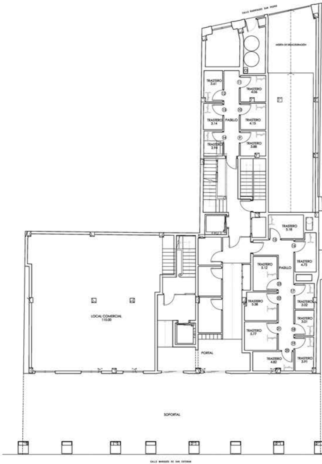
PLANTA BAJA
